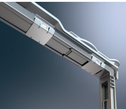
Compas d'oscillo-battant, à clipper
